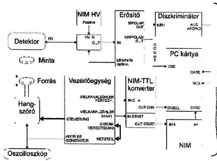
Figure 4: Mérési összeállítás
