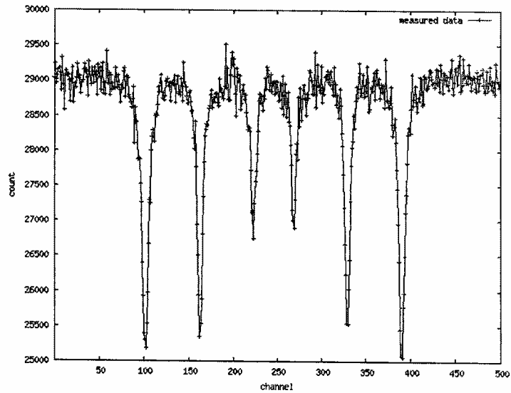
Figure 7: A negyedik feladathoz tartozó spektrum: a mágikus szög
