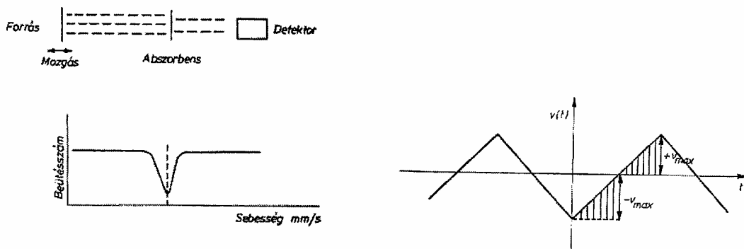
Figure 3: A mérés leegyszerűsített elvi vázlatja, valamint a forrás sebessége az idő függvényében
