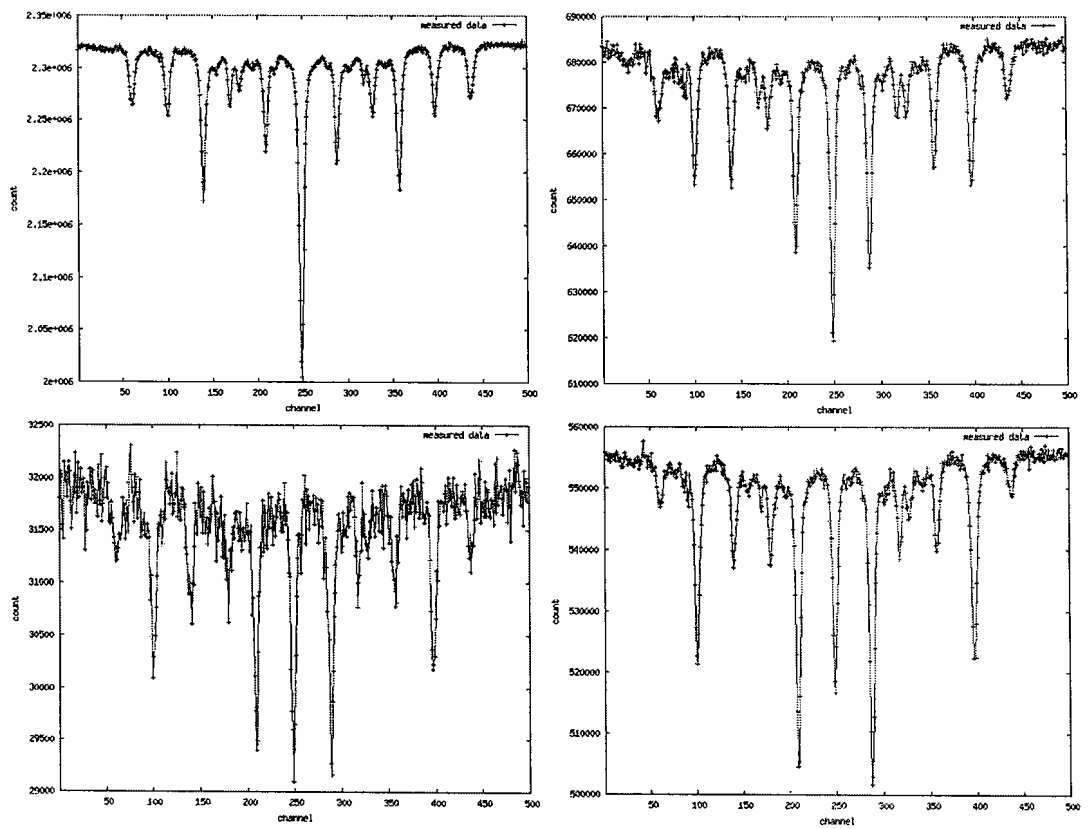
Figure 8: A különböző szögekhez tartozó spektrumok, bal felülről jobbra le: 0^\circ , 45^\circ , 60^\circ , 90^\circ
