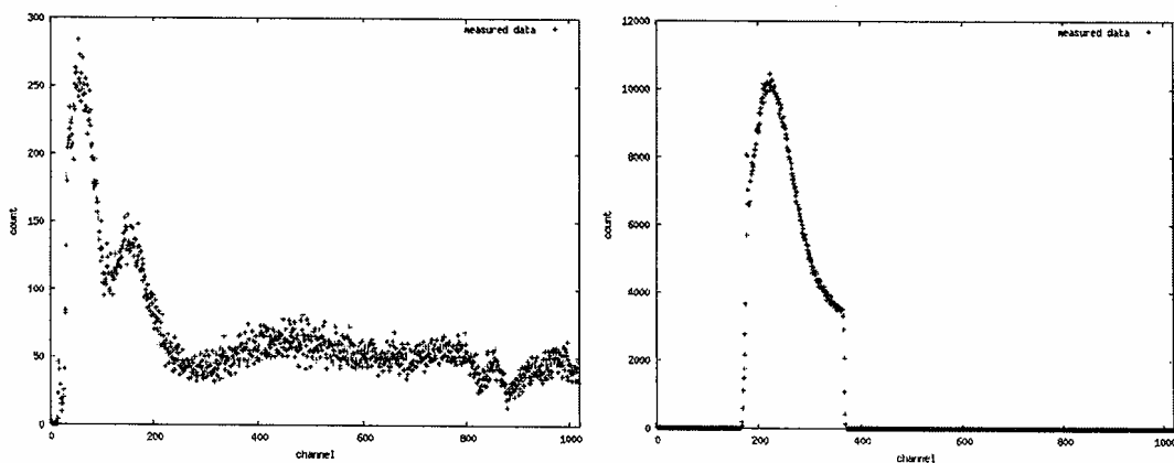
Figure 5: A teljes spektrum, valamint annak kapuzott változata
