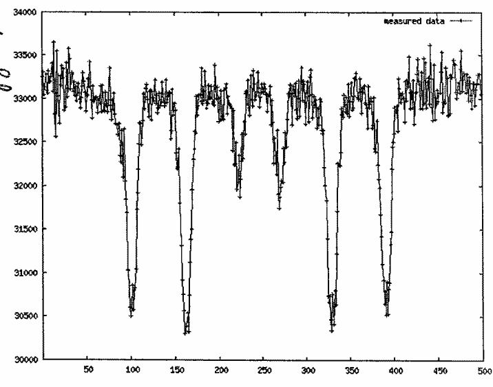
Figure 6: A harmadik feladathoz tartozó spektrum: az egysugaras merőleges spektrum
